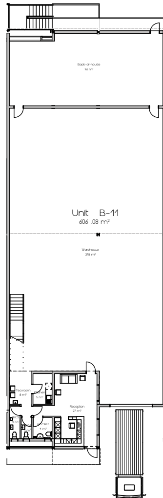
B11 Unit B11 Plan 1:200
